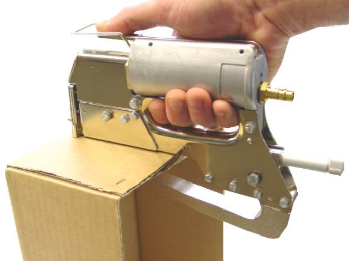
Zangenhefter pneumatisch 130/1916 P/PU/PUX | 130/2516 P/PU/PUX
